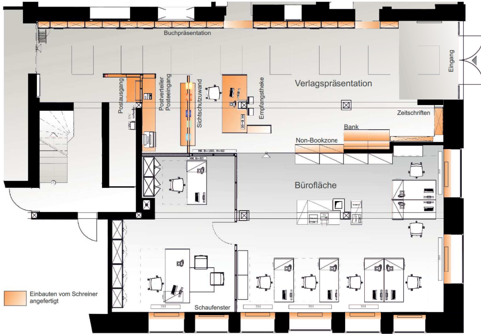
Grundriss/ Möblierungsplan - Abbildung ohne Maßstab
